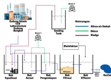
Gambar 1. Diagram Alir Proses STP di PT PLN NP UP Paiton Unit 1&2
